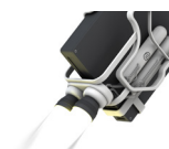
O&O Defrag
